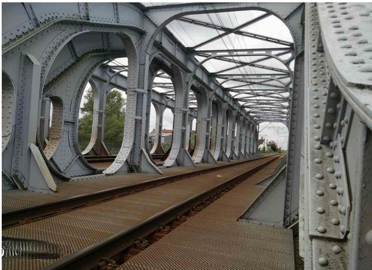
Pont Vierendeel à Grammene, près de Deinze.
